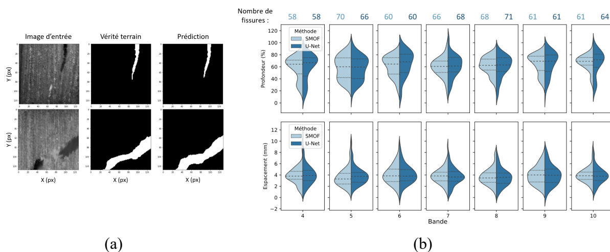
Fig. 4 : (a) Prédiction d'image du lot de test, (b) Comparaison des profondeurs et de l'espacement inter-fissures entre les fissures détectées manuellement (« SMOF ») et celle prédite par le modèle (« U-Net »)
