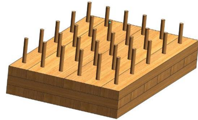
Poutres multicouches et panneaux CLT assemblés par des tourillons en bois
